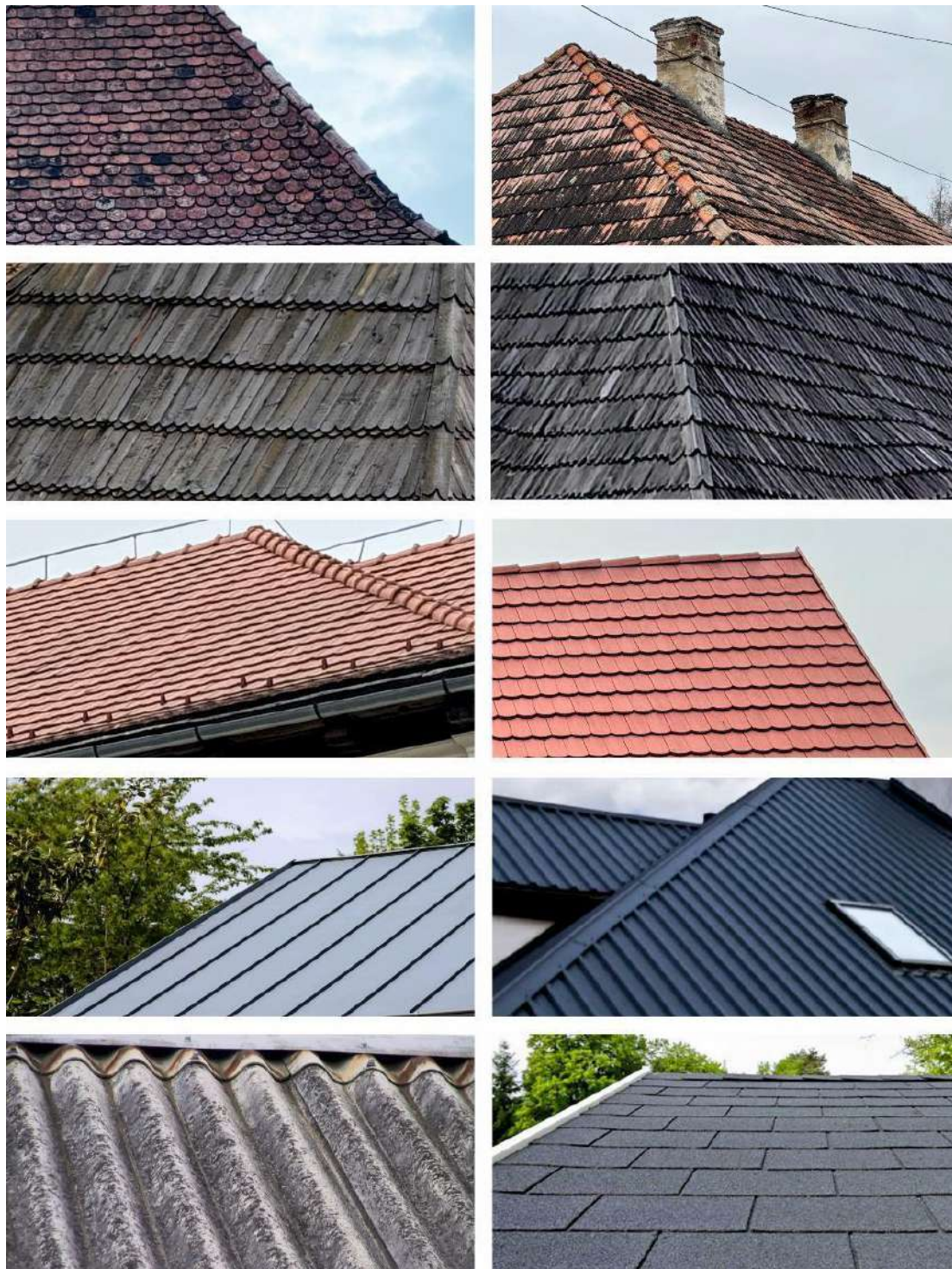
Figura 7 - Materiale permise (rândul I și rândul III – țiglă ceramică, rândul al II-lea - șită) și interzise (rândul al IV-lea - tablă cutată și rândul al V-lea - azbociment) pentru învelitorile acoperișurilor construcțiilor cu valoare ambientală, sursa: autorii Studiului Istoric General (Logic Plan SRL)
