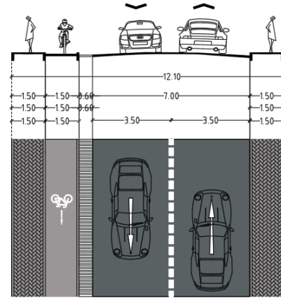
PROFIL PROPUS III-B
