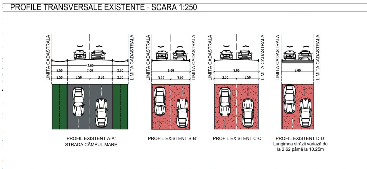
Figură 4: Profile stradale - existente
